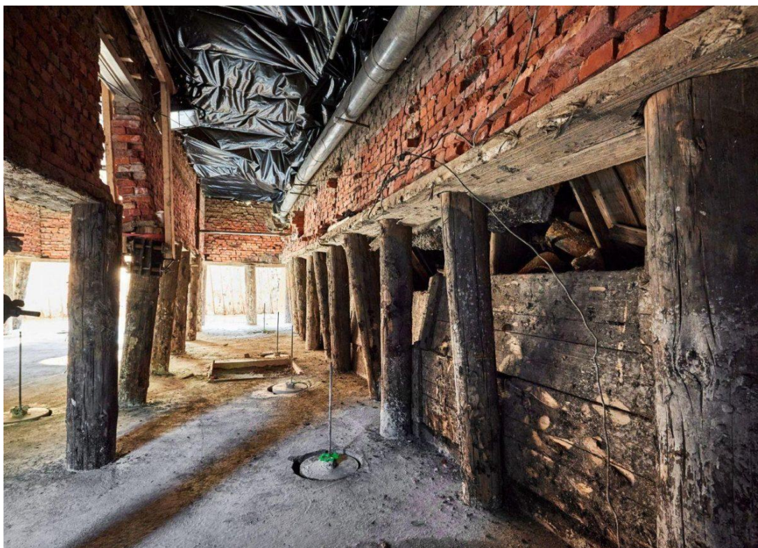
Funderingsschade door paalrot (foto Deltares)
